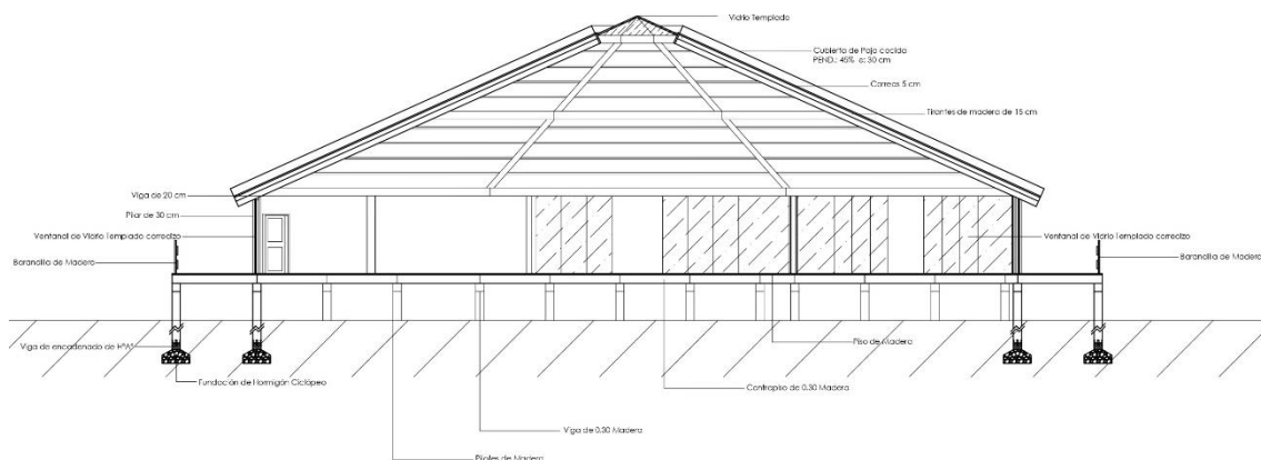
Corte AA' 3
