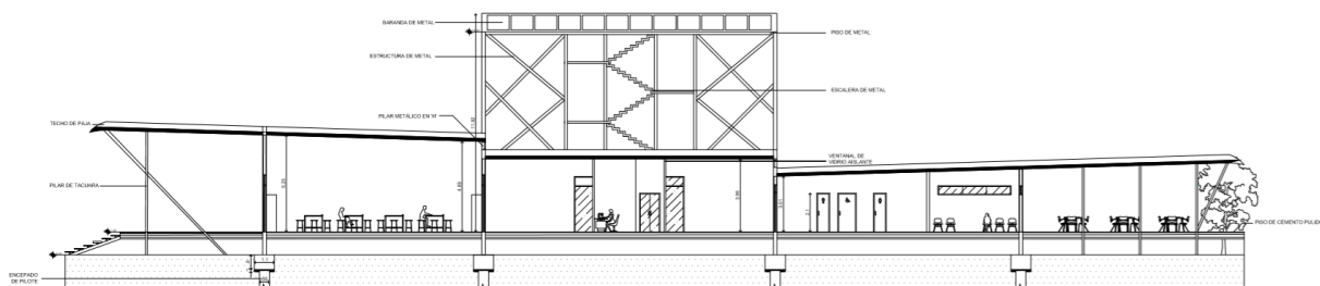
CORTE AA
