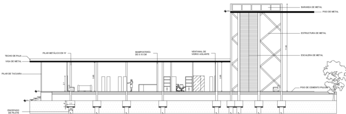
CORTE BB
